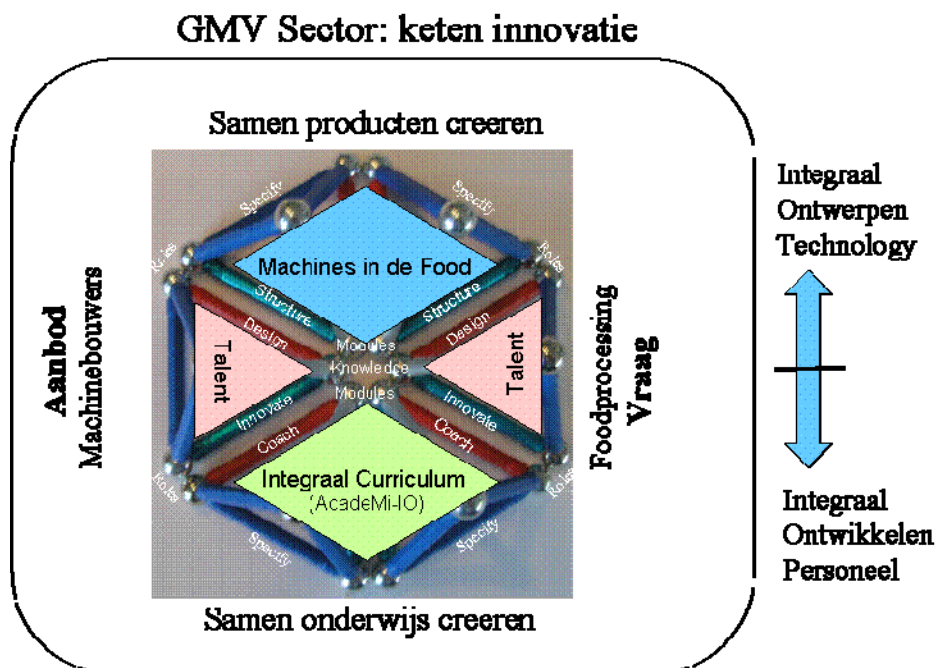
Figuur: ketendiamandmodel
