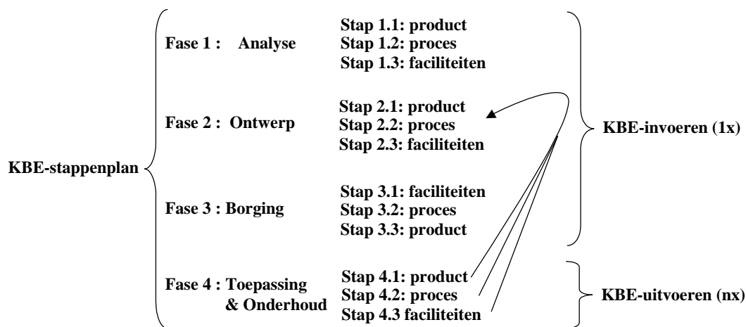
Figuur 6-1: KBE-stappenplan.
